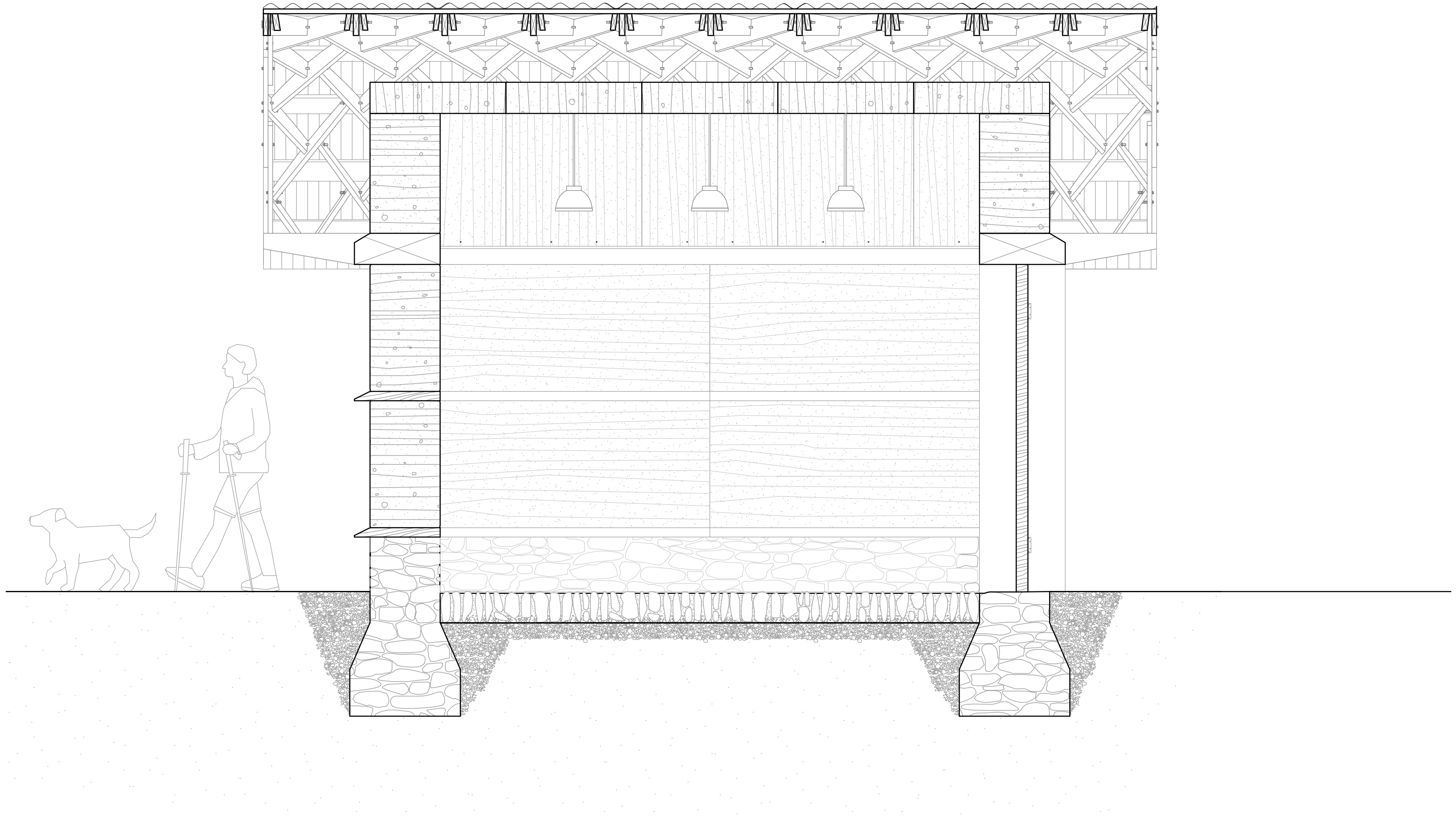
Längsschnitt
