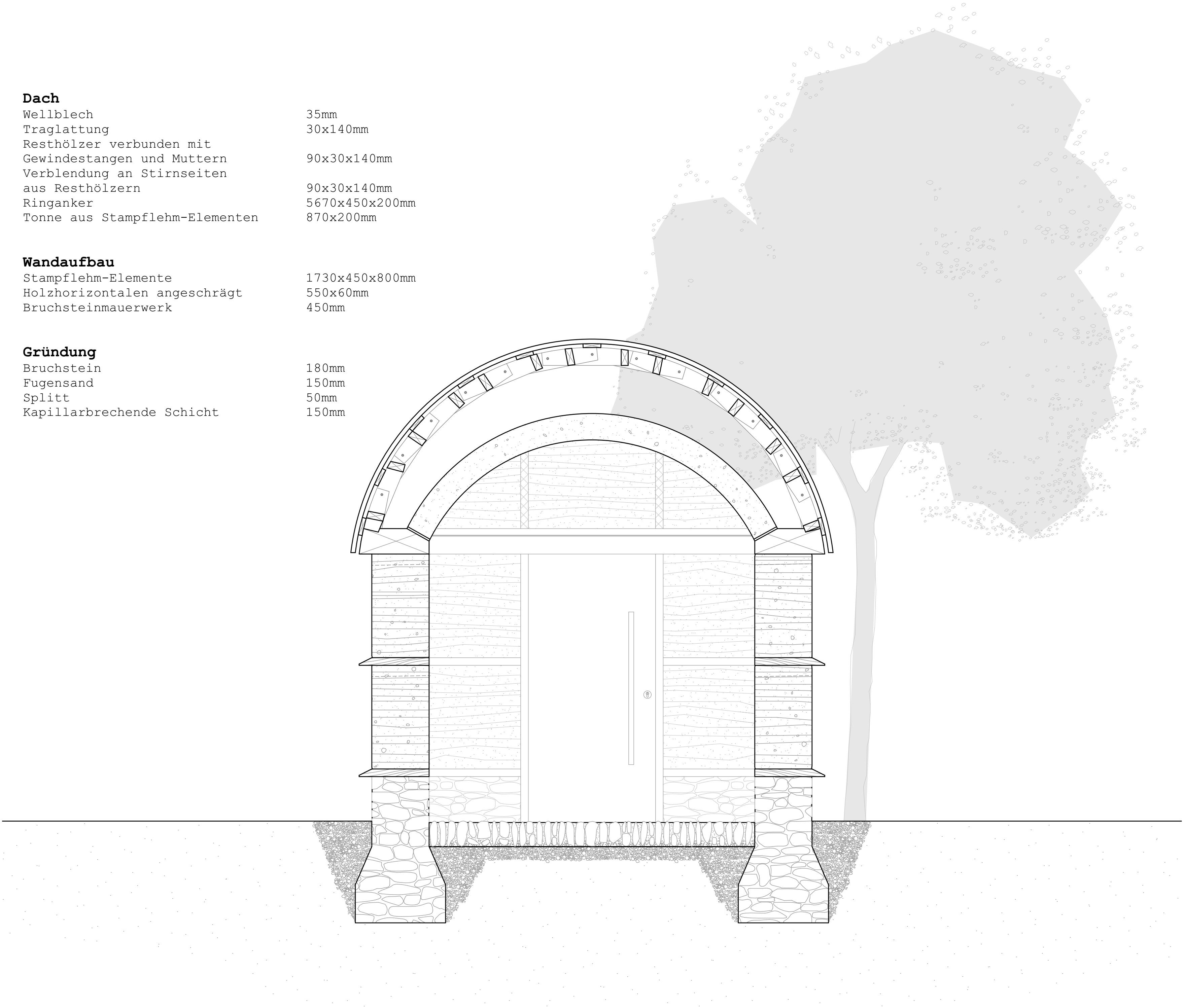
Querschnitt
