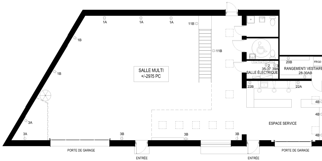
PLAN DU PLANCHER
