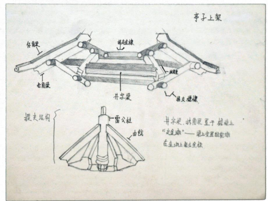
亭子结构图草稿
