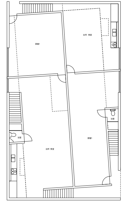
1階平面図 1:50
