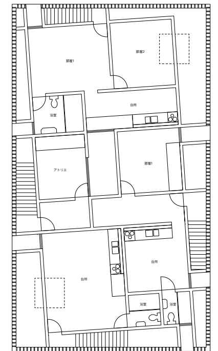
2階平面図 1:50
