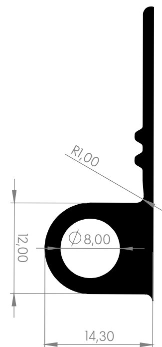
SECCIÓ B-B 2:1
