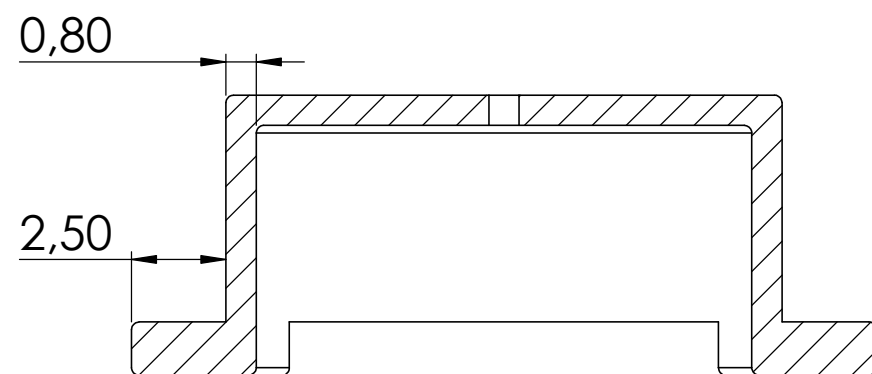
SECCIÓN W-W
