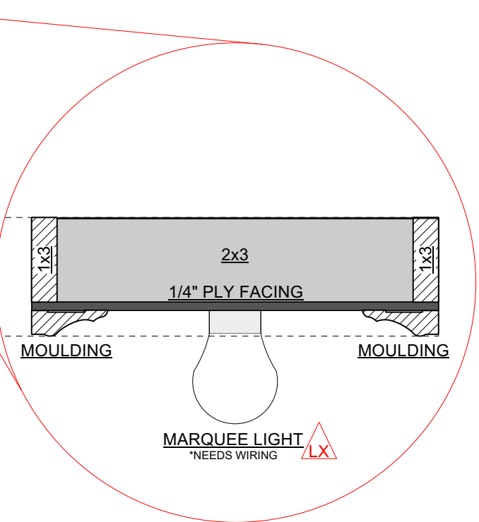
3 PROSCENIUM FRAME DETAIL Scale: 3" = 1'-0"
