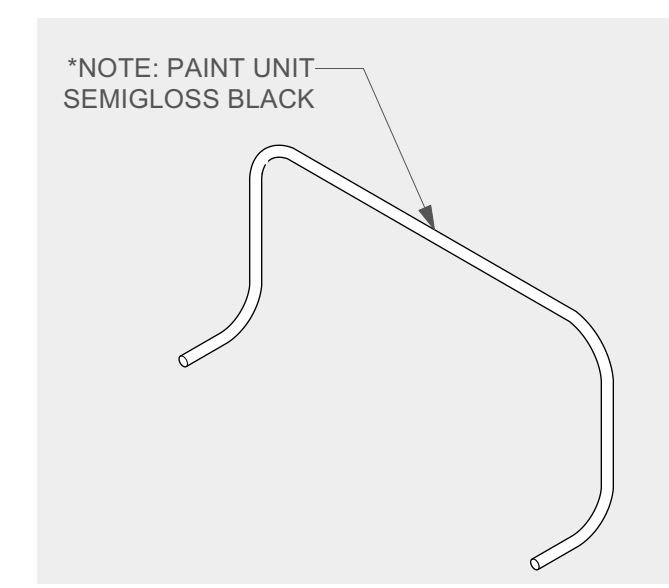
4 BENT CONDUIT ISO VIEW Scale: 1" = 1'-0"
