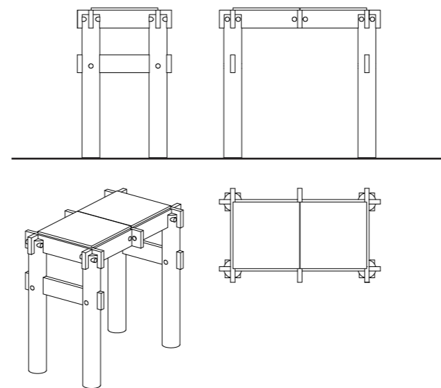
MOD.1X2.H 4x pieds 640, 5x poutres simples, 2x poutres doubles, 12x tourillons, 2x plaques
