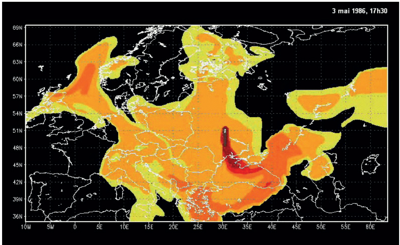
Concentration du césium 137 dans l'air au dessus du sol après Tchernobyl, Bq/m 3 Source : IRSN
